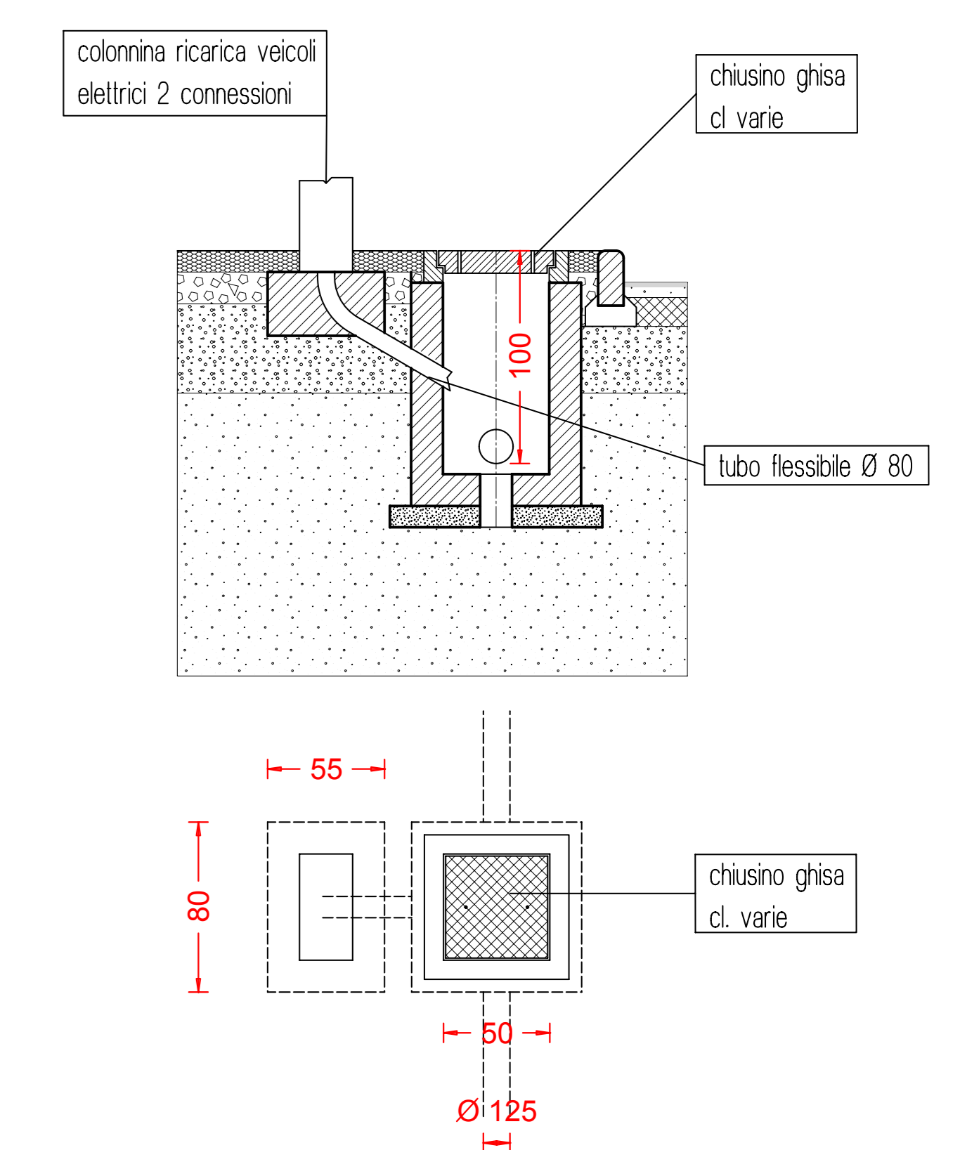
PARTICOLARE COLONNINA RICARICA AUTOVEICOLI ELETTRICI scala 1:25
