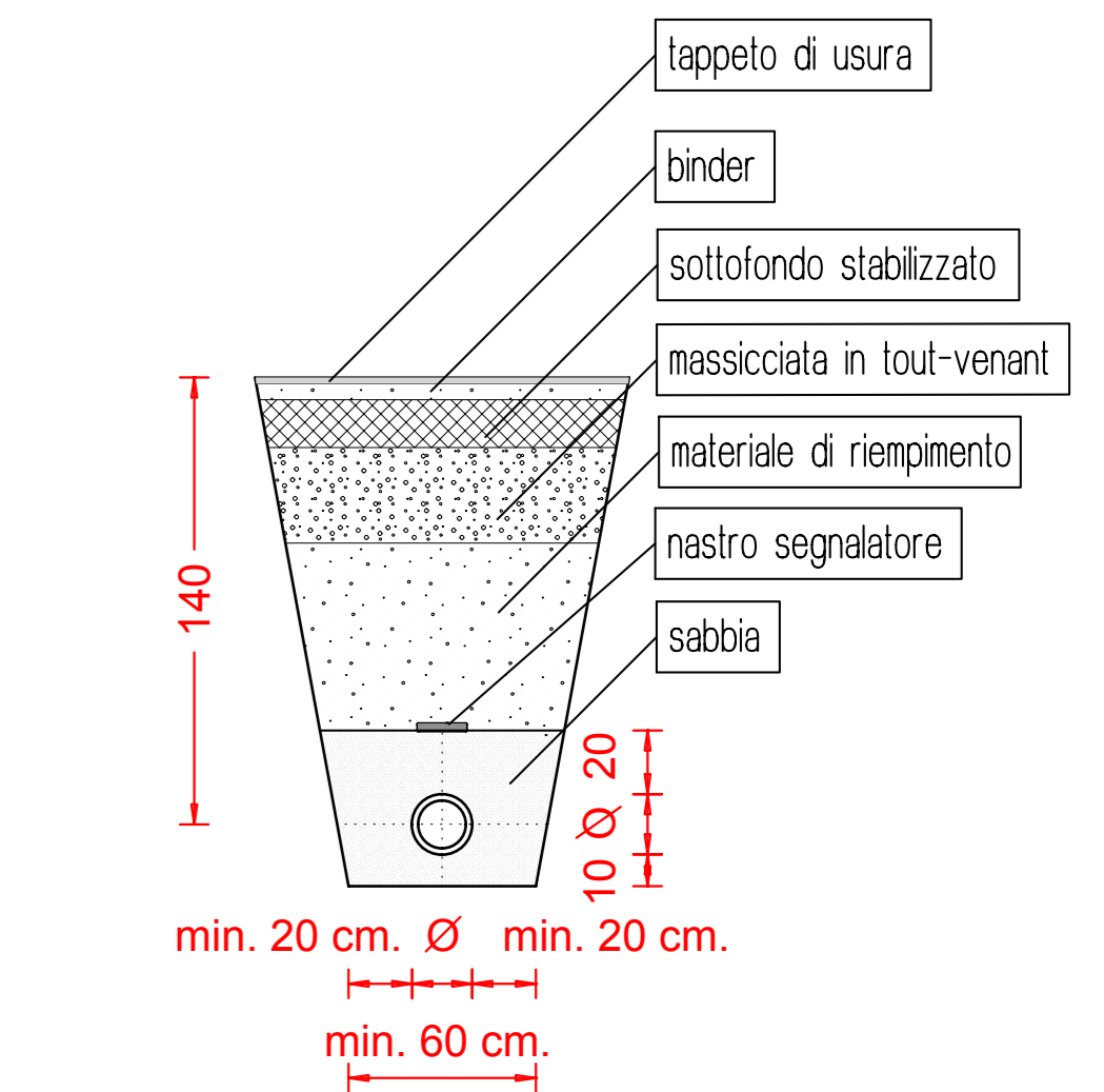
PARTICOLARE POSA CONDotta ACQUEDOTTO scala 1:25
