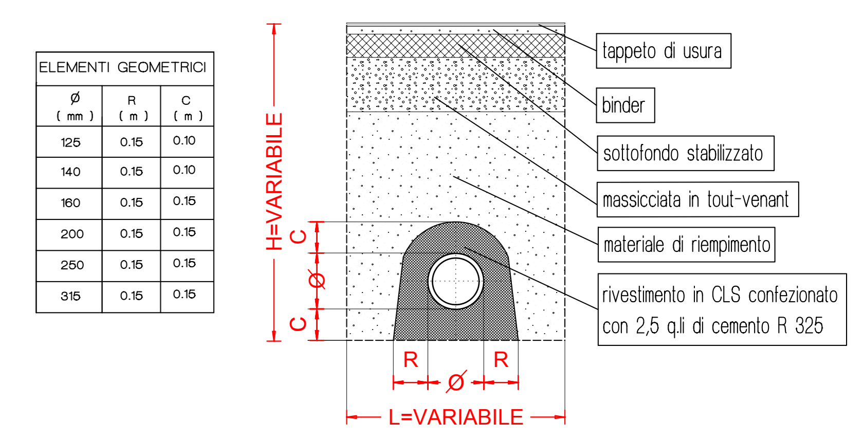
PARTICOLARE POSA CAIVODOTTI scala 1:25
